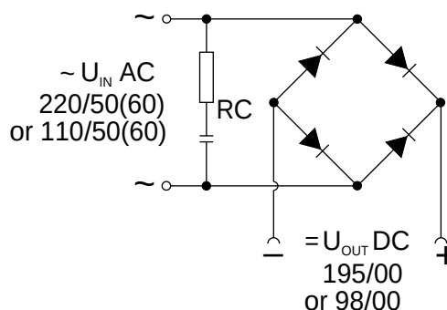
rectifier scheme
